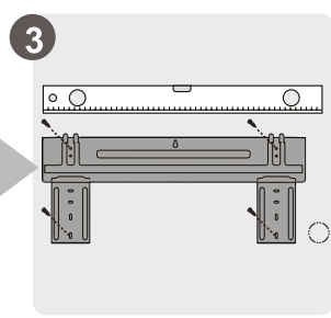
Инсталиране на монтажната основа
